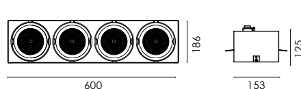
MODO FRAMELESS 4 LIGHT
